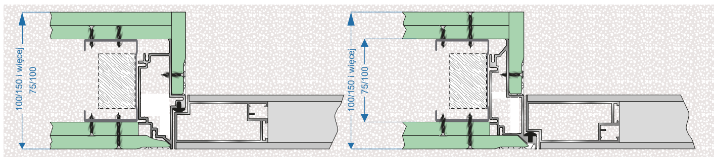
Rys. 6 – MONTAŻ OŚCIEŻNICY W ŚCIANIE G-K
