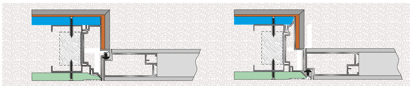
Rys. 8 – OBRÓBKĄ OŚCIEŻNICY PŁYTKĄ CERAMICZNĄ
