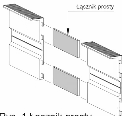
Rys. 1 Łącznik prosty do listew cokołowych
