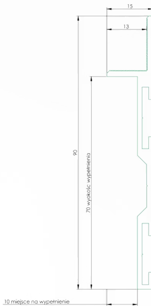
Rys. 2 – Listwa Zeromur do ściany murowanej
