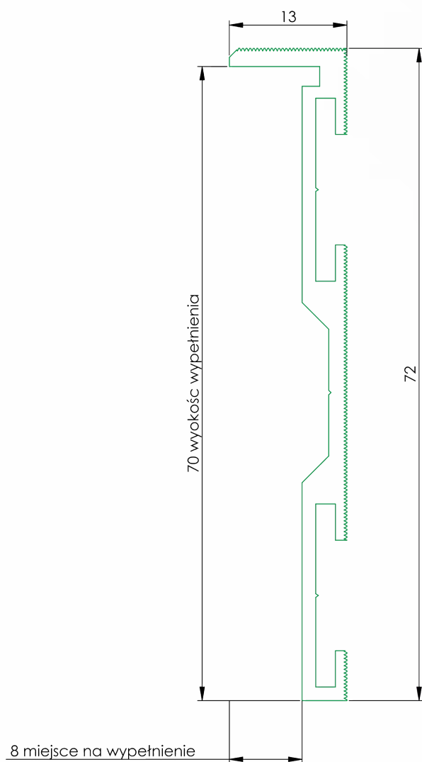
Rys. 1 – Listwa Zeromur do gips-karton
